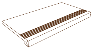
Bordo costa retta con incisioni Linear bevelled straight edge coping Linearer Rand mit gerader Kante Nez de marche linéaire Borde canto recto lineal 60x30x4 24"x12"x2"
