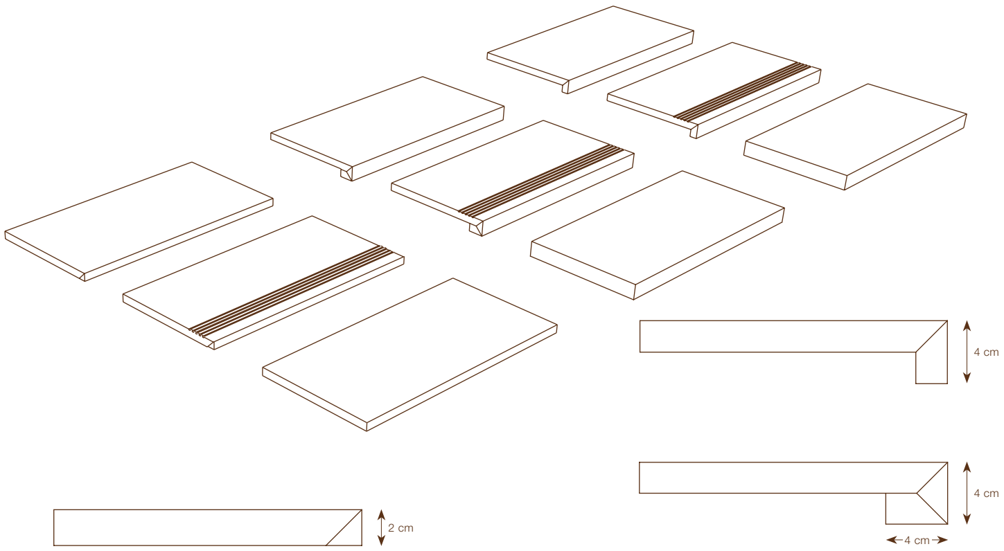
Bordo costa retta lineare Linear bevelled straight edge coping Linearer Rand mit gerader Kante Nez de marche linéaire Borde canto recto lineal 60x30x4 24"x12"x2"
